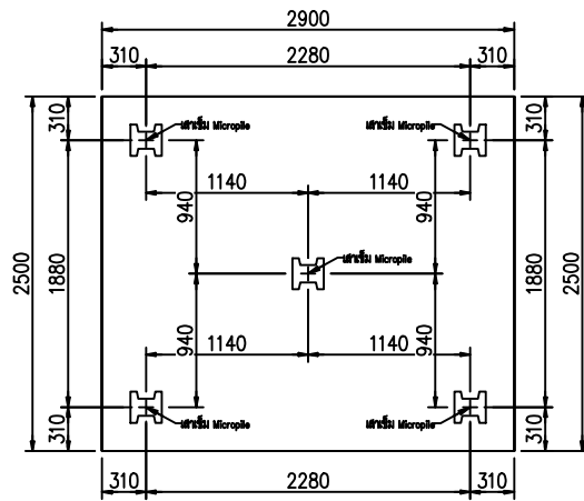
ตำแหน่งเสาเข็ม
