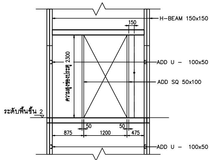
แบบประตูหน้าต่างชั้น 2
