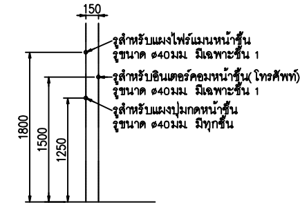
แบบระยาระเบียงคดหน้าชั้น
