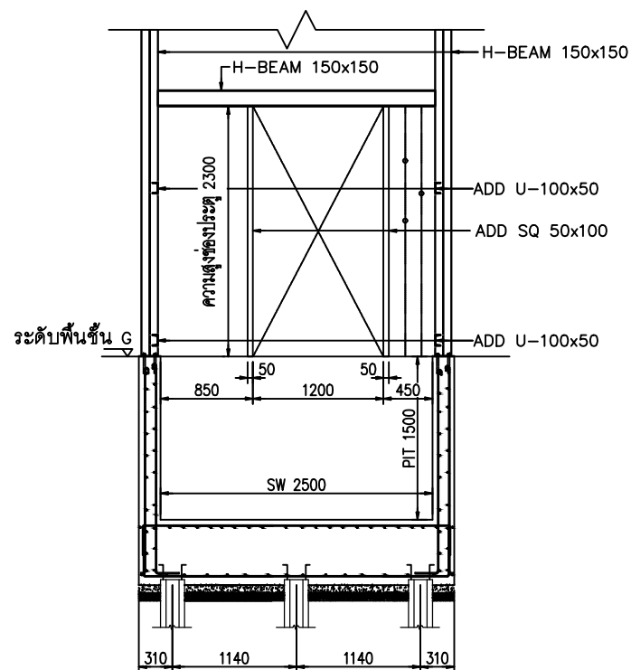
แบบประตูหน้าต่างชั้น G
