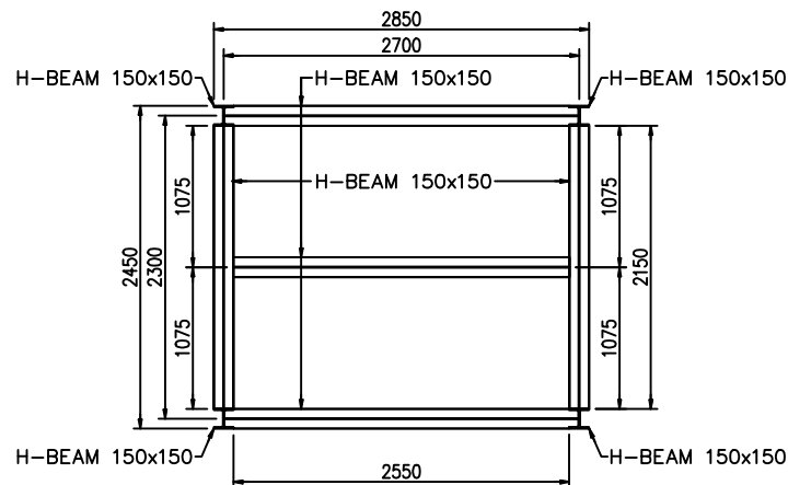
แบบคานหลังคาปล่องลิฟต์
