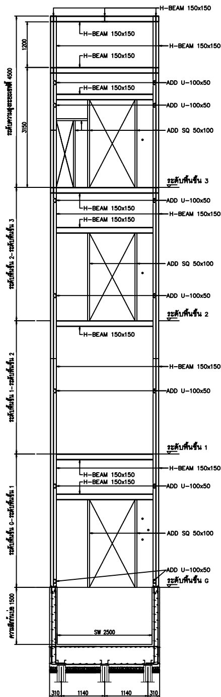
แบบตัดด้านหน้า
