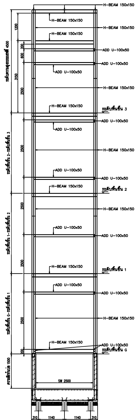
แบบตัดด้านหลัง
