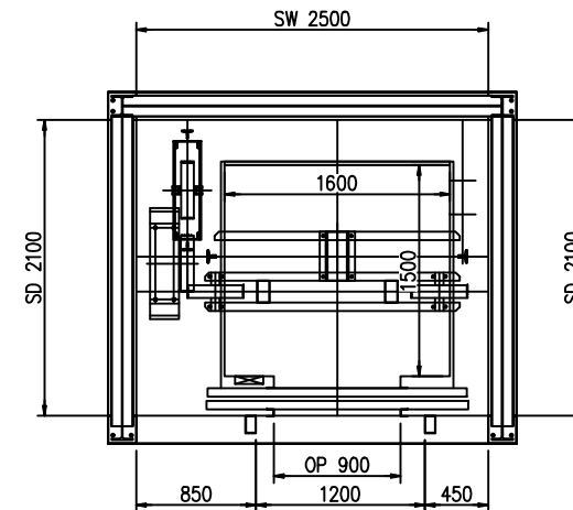
แบบติดตั้งลิฟต์
