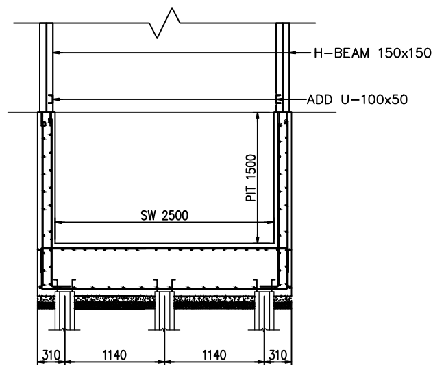
รูปตัดบ่อลิฟต์
