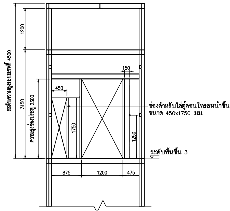
แบบประตูหน้าชั้น 3
