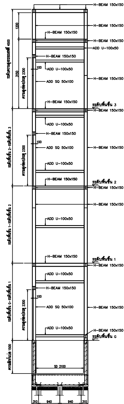
แบบตัดด้านข้าง
