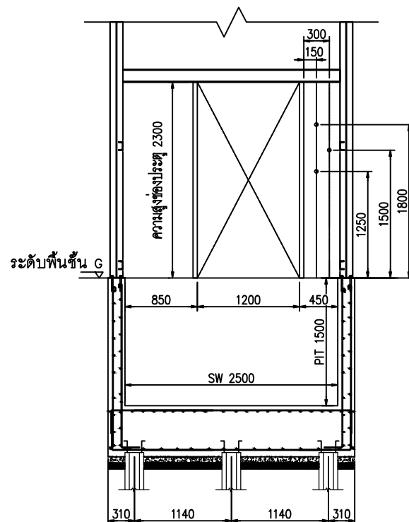
แบบประตูหน้าชั้น G
