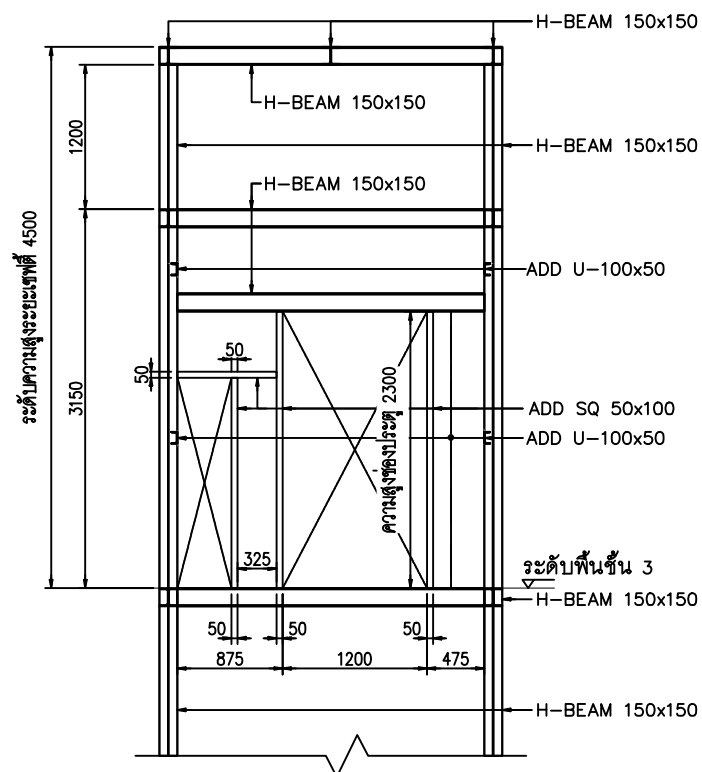
แบบประตูหน้าต่างชั้น 3
