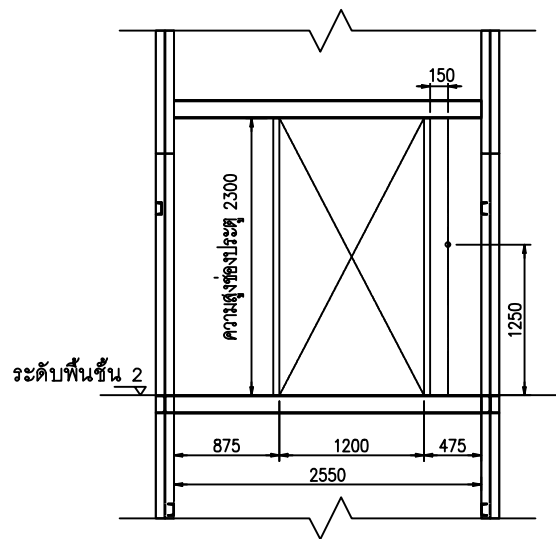
แบบประตูหน้าชั้น 2
